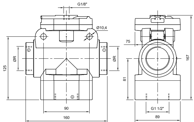
AZ 7 - Comando pneumático
