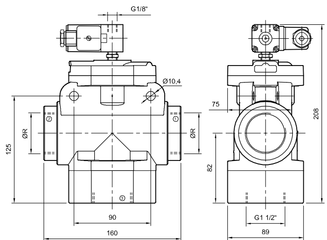
AZ 7 - Comando eletropneumático (30 bar)
