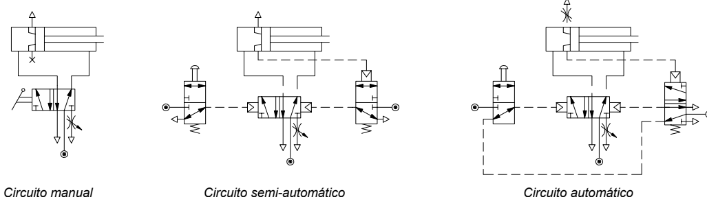
Circuito manual
